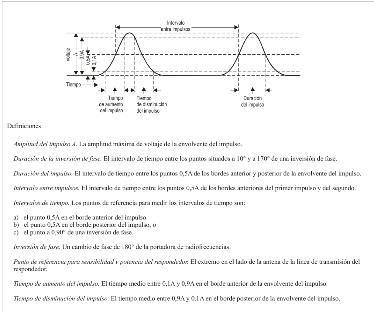
Figura 3-1. Definiciones de las formas de ondas, intervalos y puntos de referencia para sensibilidad y potencia del radar secundario de vigilancia
