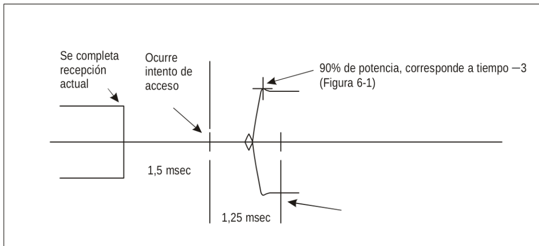
Figura 6-3. Tiempo de actuación de recepción a transmisión
